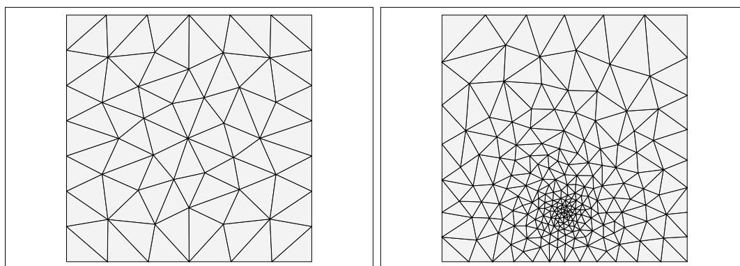
(a) Maillage uniforme (b) Concentration ponctuelle
