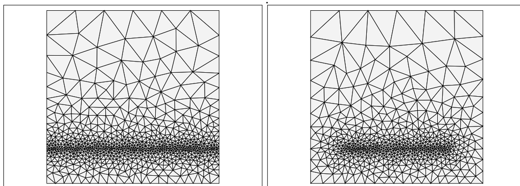
(a) Concentration axiale (b) Concentration sur un segment
